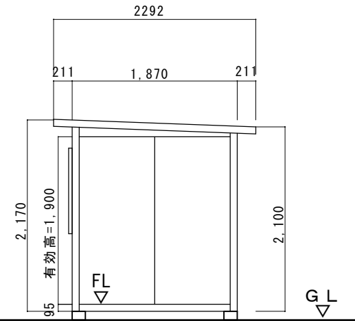
【C立面図】
