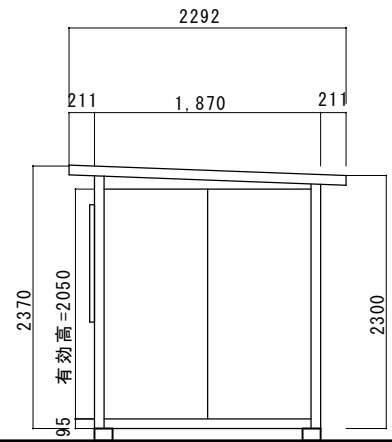
【D 立面図】
