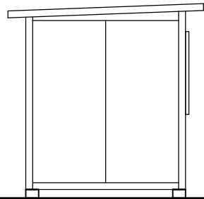
【B 立面図】
