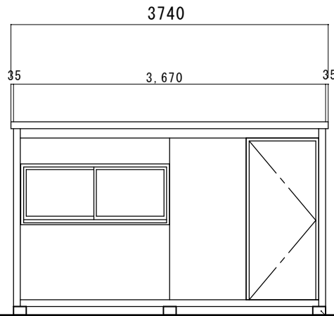
【A 立面図】
