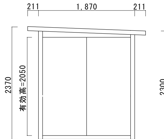
【立面図】
