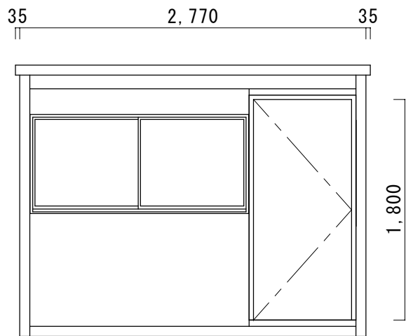
【立面図】
